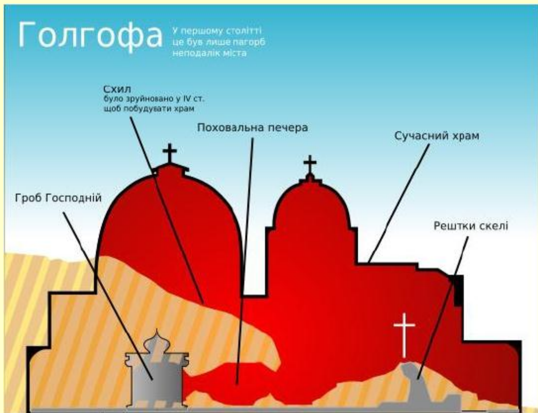
Загальна схема Храму Гробу Господнього
